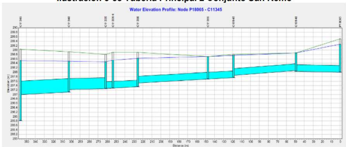
Ilustración 5-38 Tubería Principal 2 Conjunto San Remo
